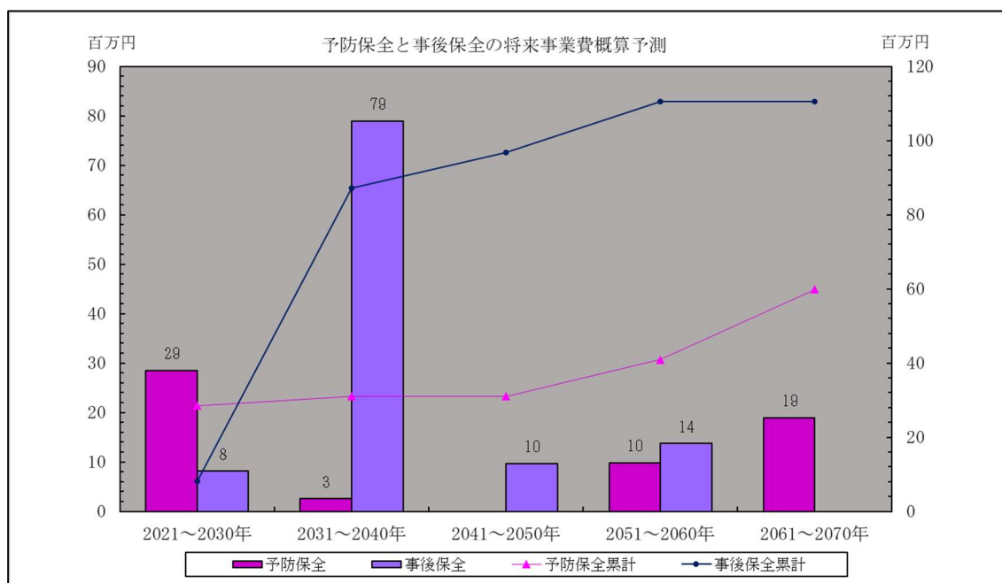
図6-1 50年間の維持管理の比較試算結果
