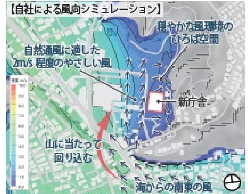
【図5-3: 周辺環境による敷地の風向き】
