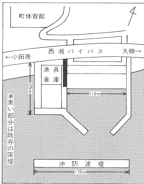
二宮漁港の基本計画
