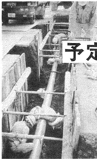
公共下水道工事(開削工法)
