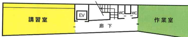
2階平面図
