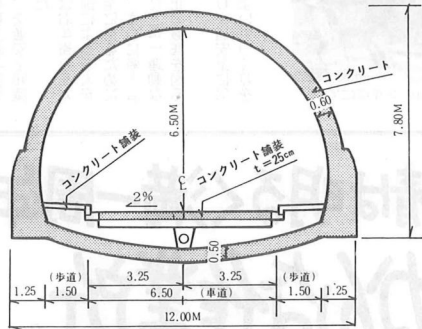
トンネル内標準断面図
