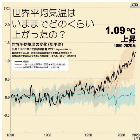
図4 世界平均気温の変化（1850年～2020年・観測）
