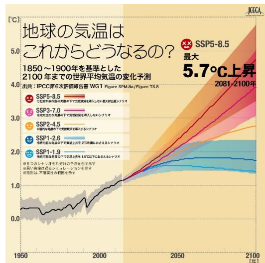
図5 世界平均気温の変化予測（観測と予測）
